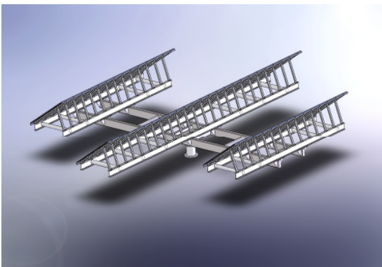
einachsig nachgeführte Solaranlage
